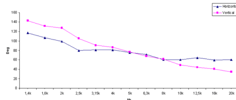
BEAMWIDTH
